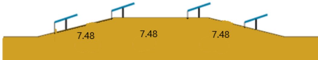
Fig.4 Distanca e paraparë mes strukturave montuese te PV moduleve
