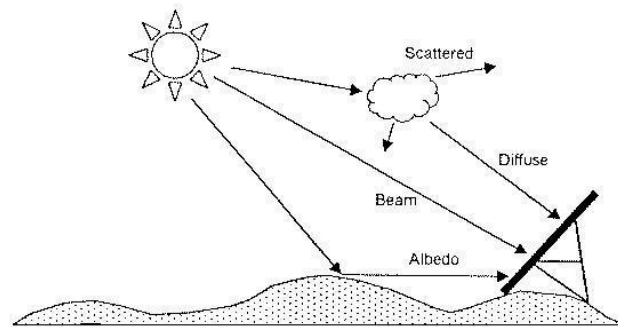
Fig.9 Rrezet nga rrezatimi diellor
