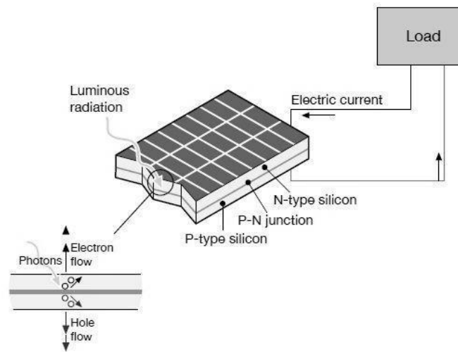
Fig.7 Parimi i punës së qelizave fotovoltaike
