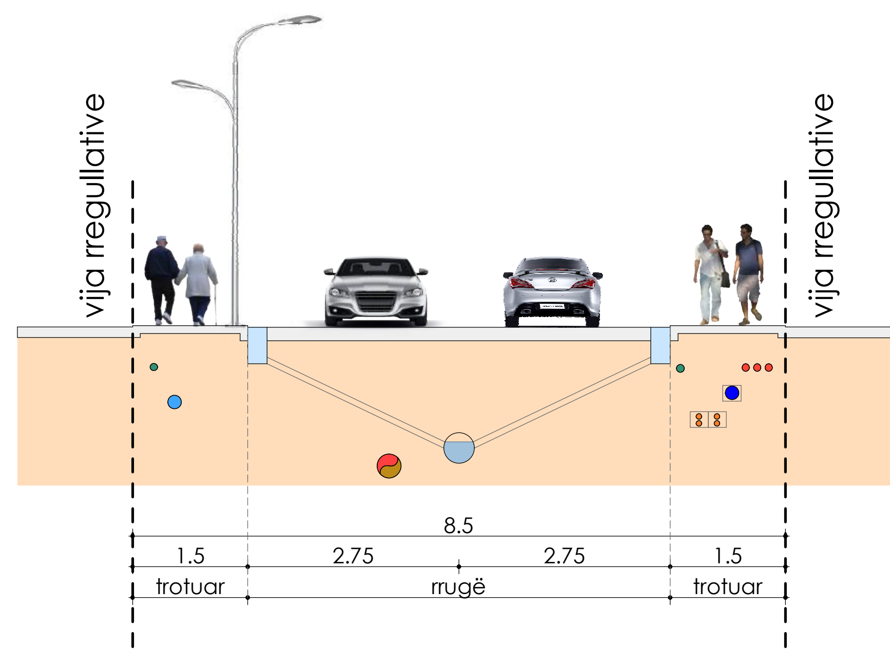
RRUGË LOKALE 3-3
