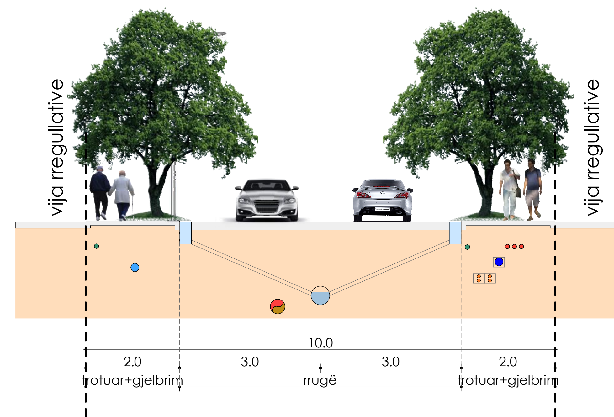
RRUGË PËRMBLEDHËSE 2-2
