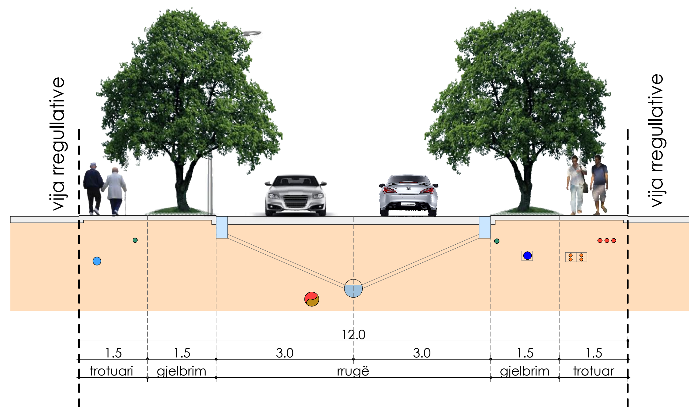
RRUGË PËRMBLEDHËSE 1-1
